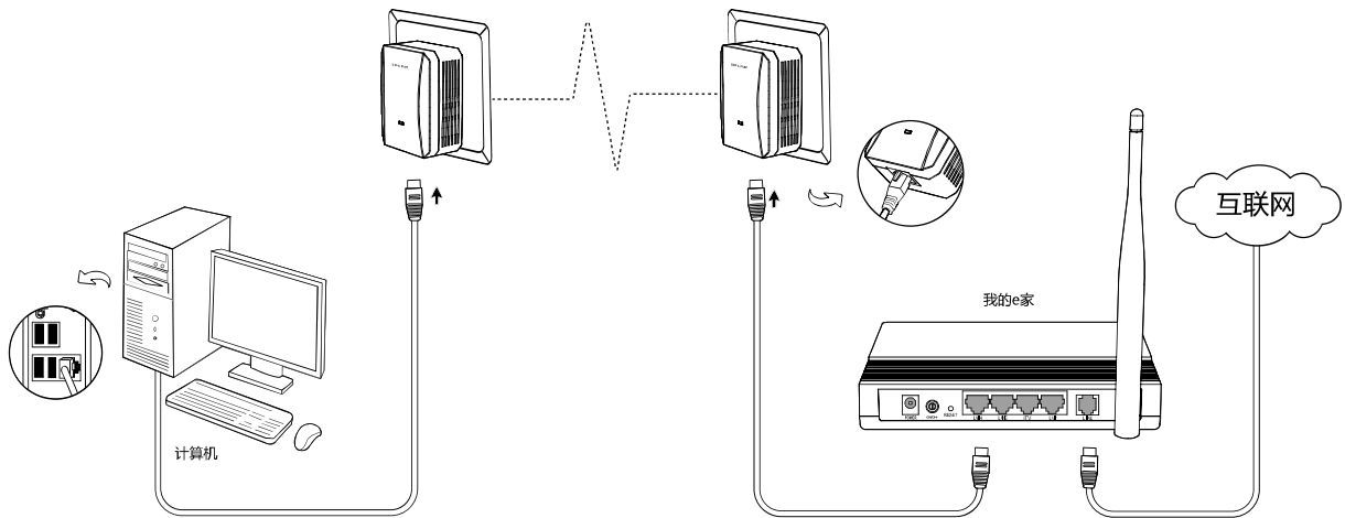
图2-4 整体连接图
